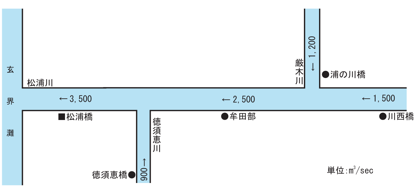
松浦川計画高水流量図
