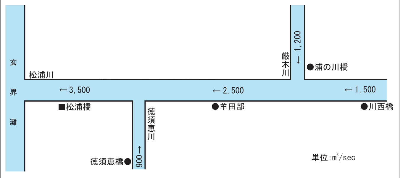
松浦川計画高水流量図
