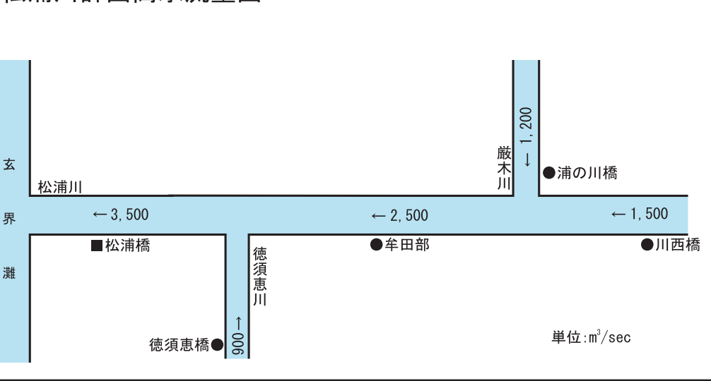
松浦川計画高水流量図
