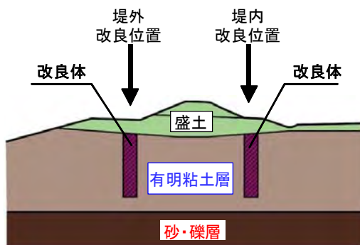
図 1.2.9 軟弱地盤上の築堤イメージ
