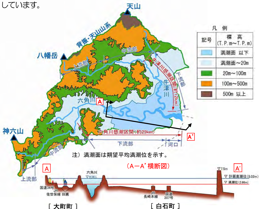
図 1.1.2 六角川流域内標高及び地形横断面
