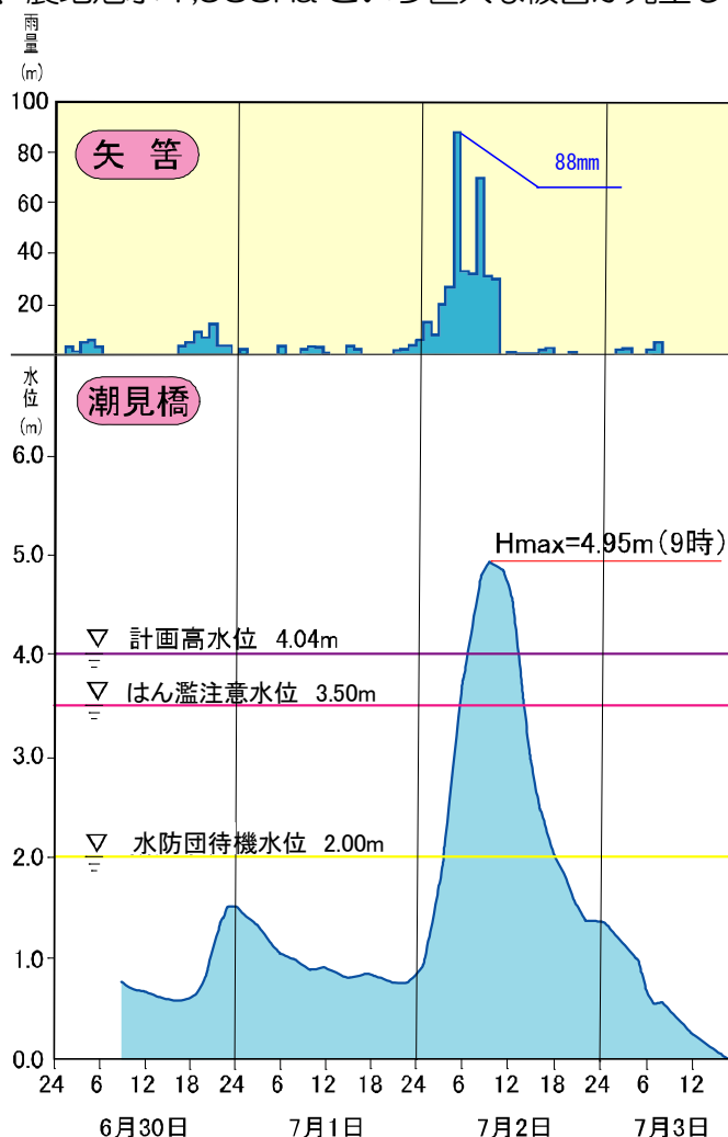
図 1.2.2 六角川洪水状況図
