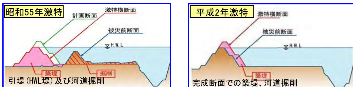
図 1.2.8 2度にわたる激特事業での河川改修イメージ
