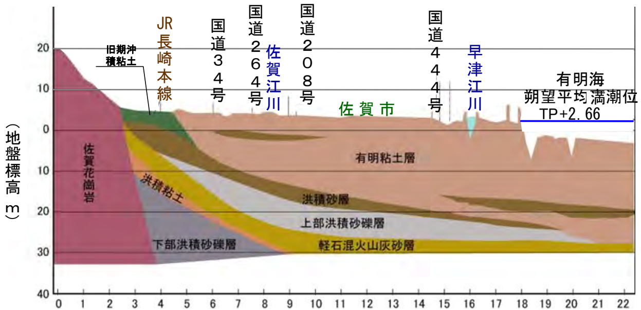
図 1.1.7 佐賀平野地質横断図
