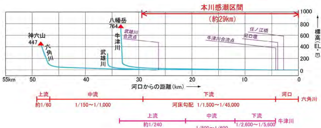
図 1.1.3 六角川本支川縦断面
