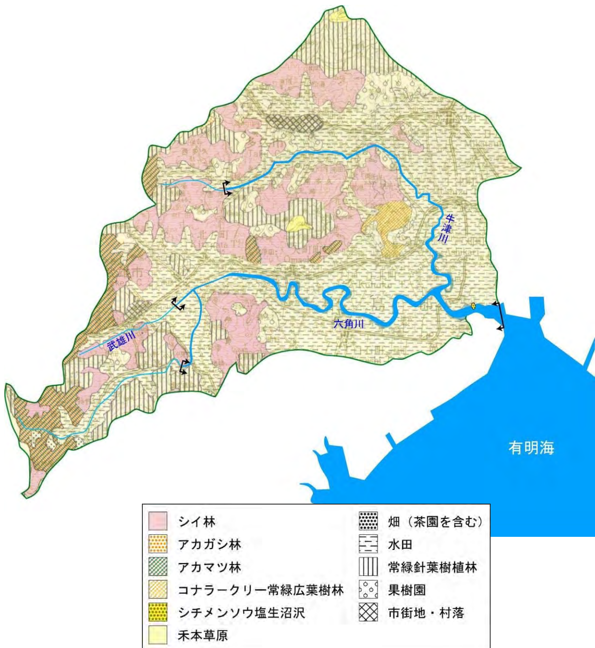
図 1.1.12 六角川流域植生図 (出典：佐賀県植生図)
