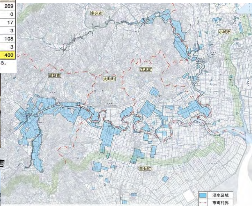
図 1.2.4 浸水区域図（平成 21 年 7 月洪水 市別聞き取り調査および武雄河川事務所内水痕跡調査による）
