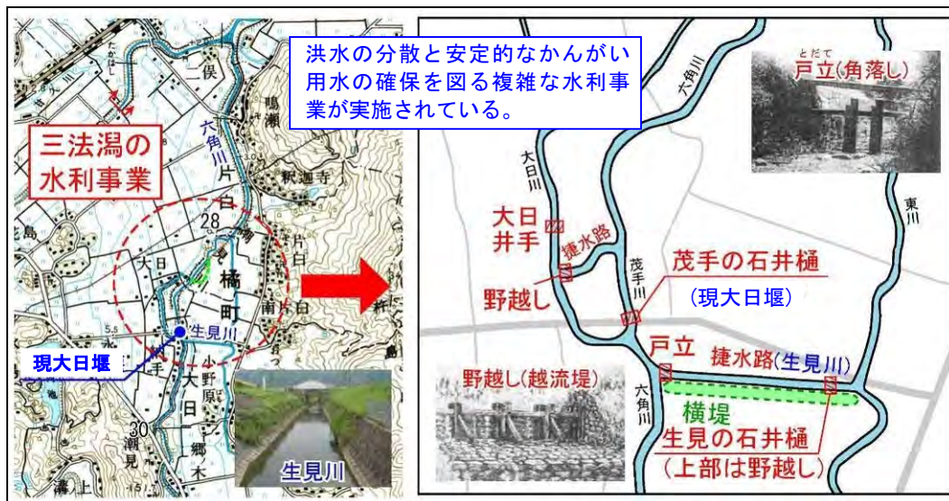
図 1.2.5 成富兵庫茂安による三法湯の水利事業（寛永 2 年(1625) 竣工）
