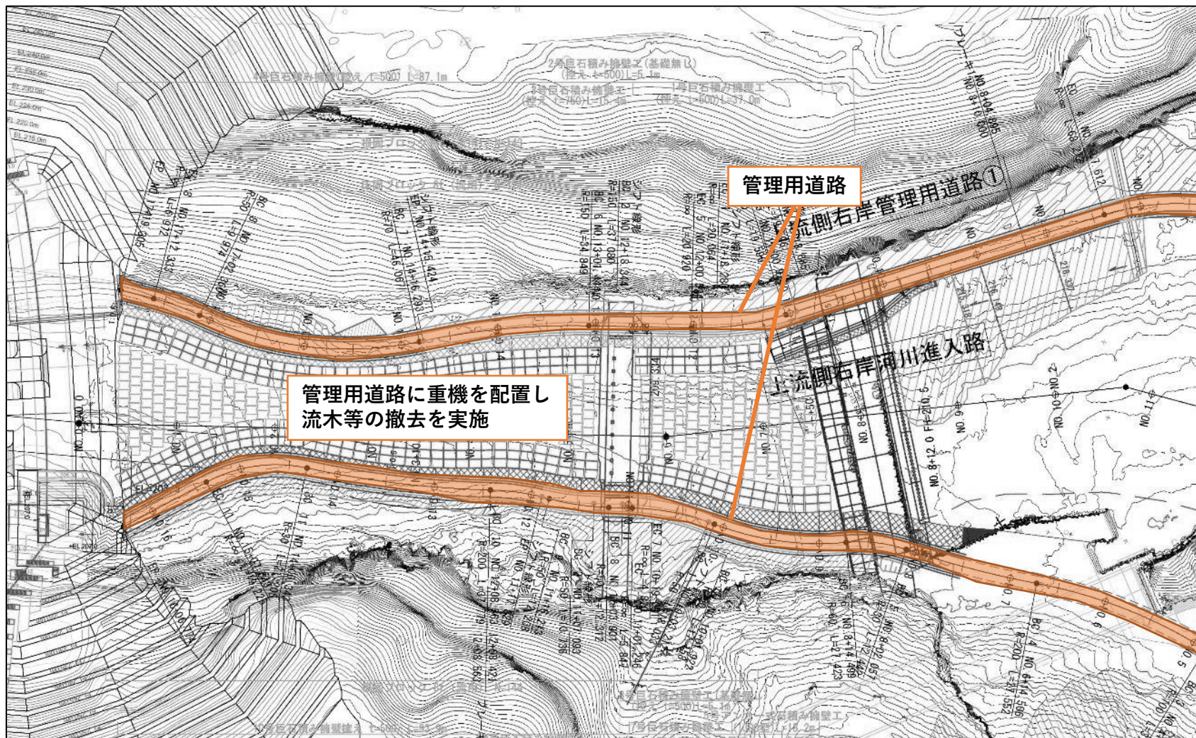
図-1 管理用道路計画図
