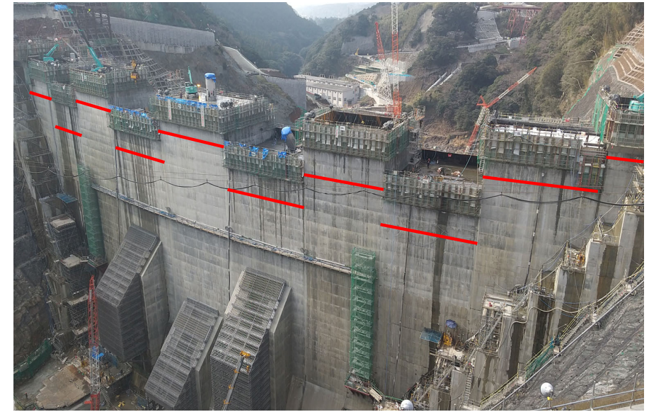
令和4年12月末時点（赤線より上部を打設）
