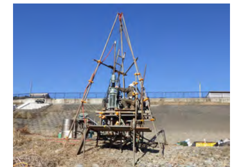
地質調査の状況（R5.2.23） 【球磨村渡地区（引堤）】
