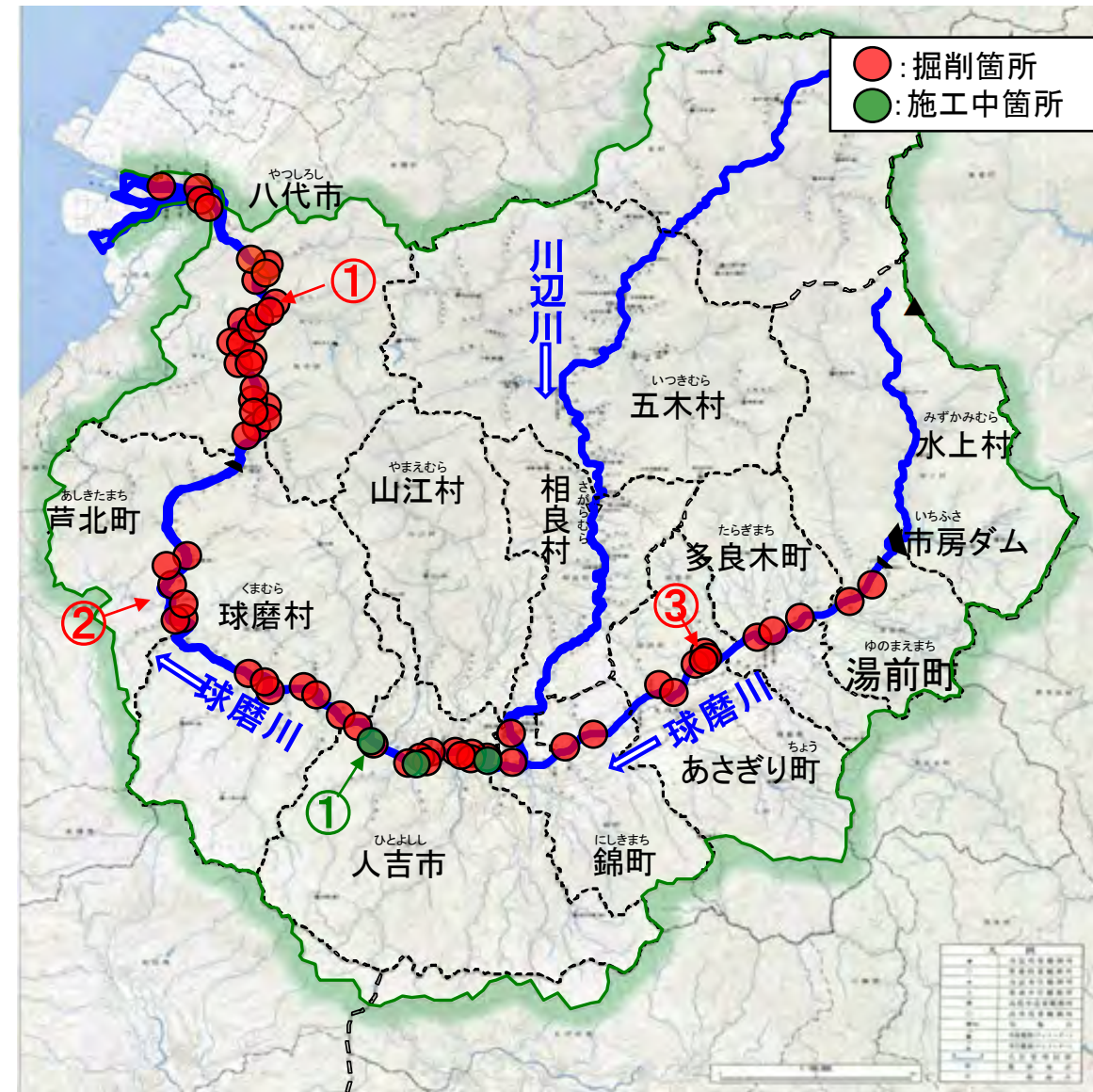
【施工中状況】
